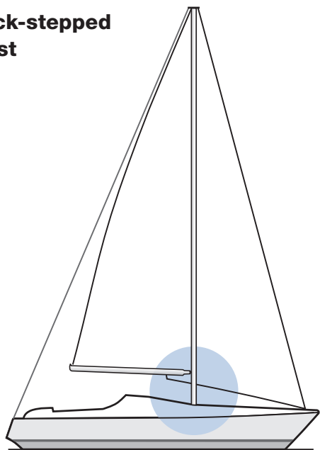
Keel-stepped mast
